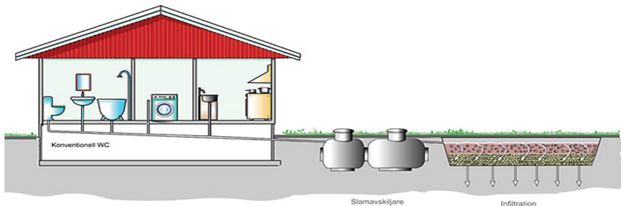
Bild: Principskiss för infiltration ( www.avloppsguiden.se )
