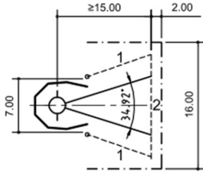
Figur 2 – Exempel på kastbur. (IAAF Track and Field Facilities Manual, 2008) [4]
